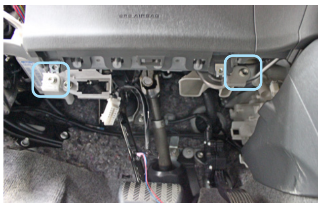
Фото 1.11. Болты крепления подушки безопасности
